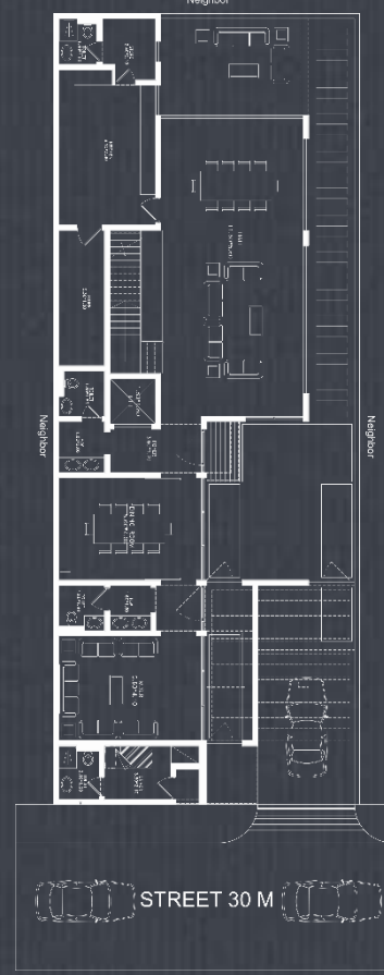
الدور الارضي
